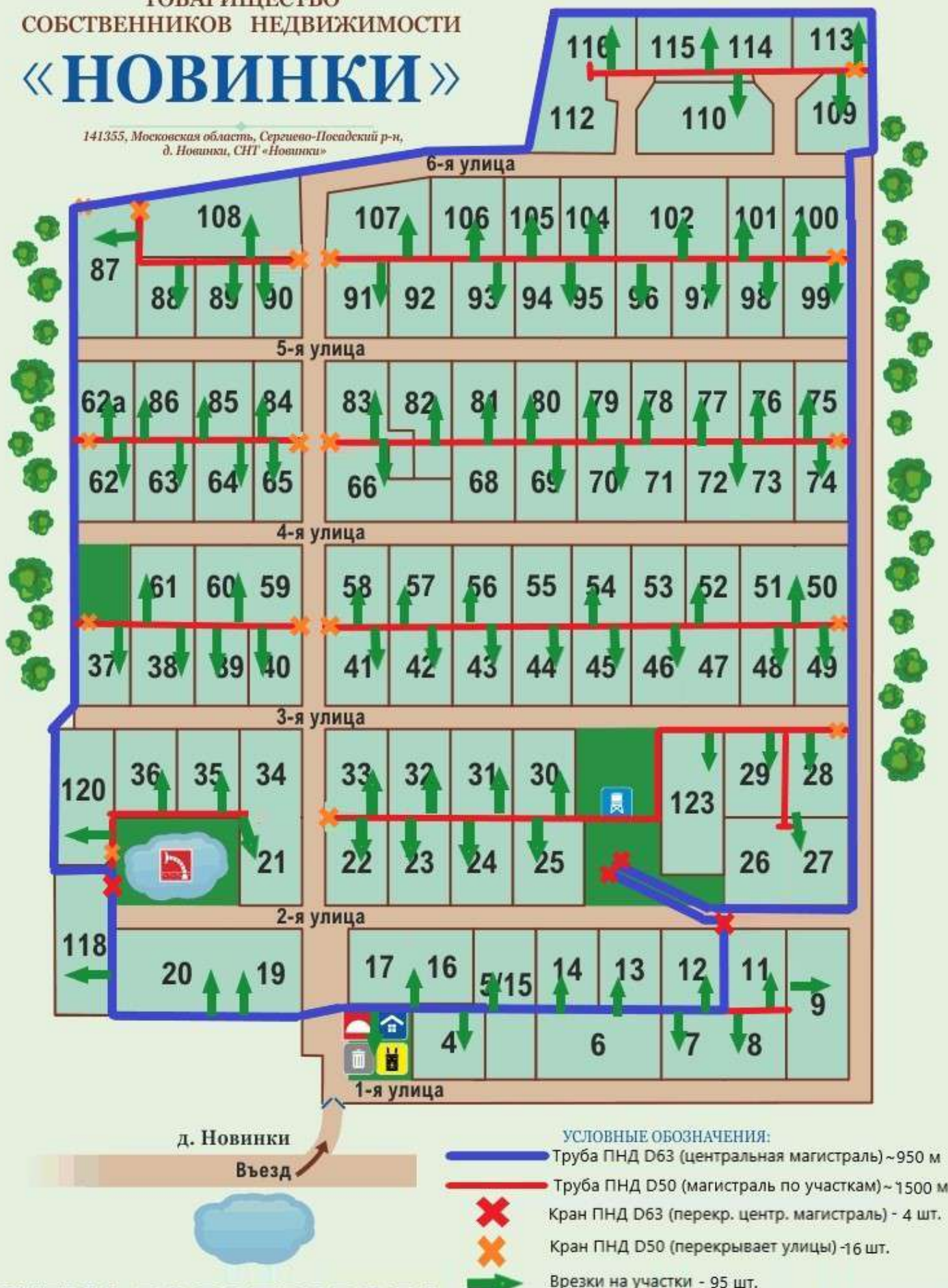
СХЕМА ВОДОПРОВОДА
